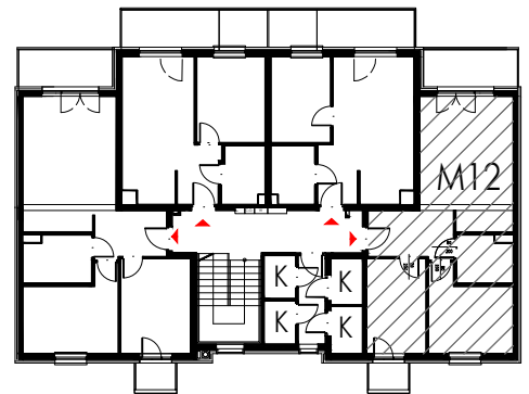
RZUT KONDYGNACJI
